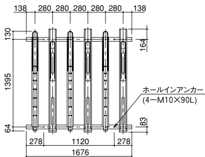
CFB-286 平面図
