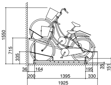
側面図
