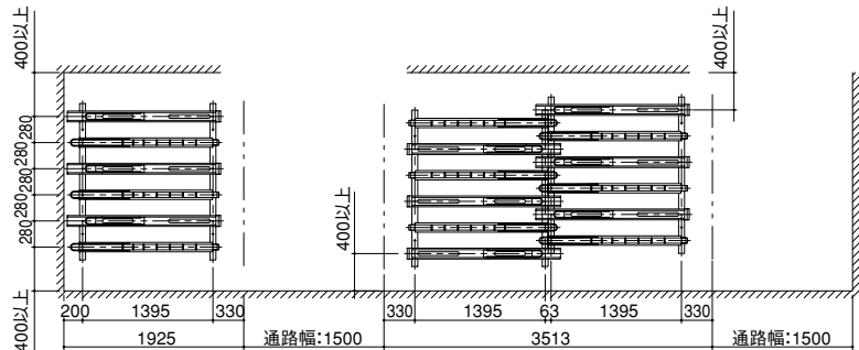
直角配列 配置例
