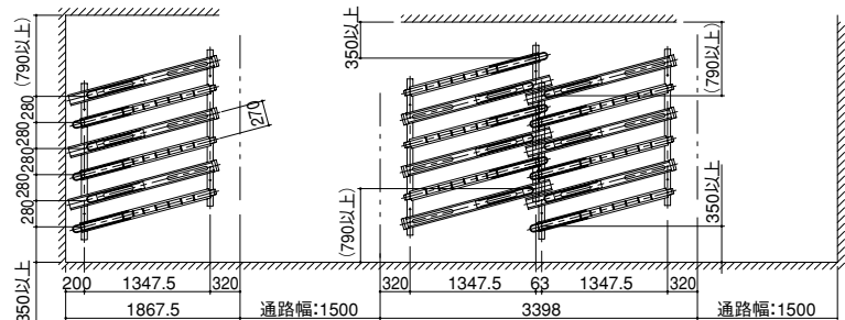
15°斜め配列 配置例
