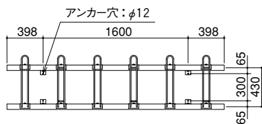
CRSB-406 平面図
