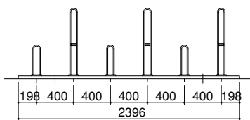
CRSB-406 正面図
