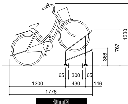
側面図
