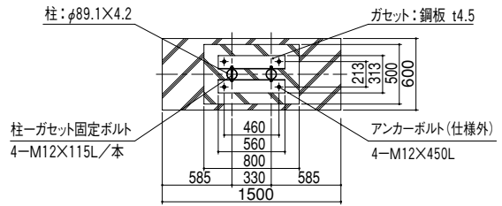
基礎部平面図
