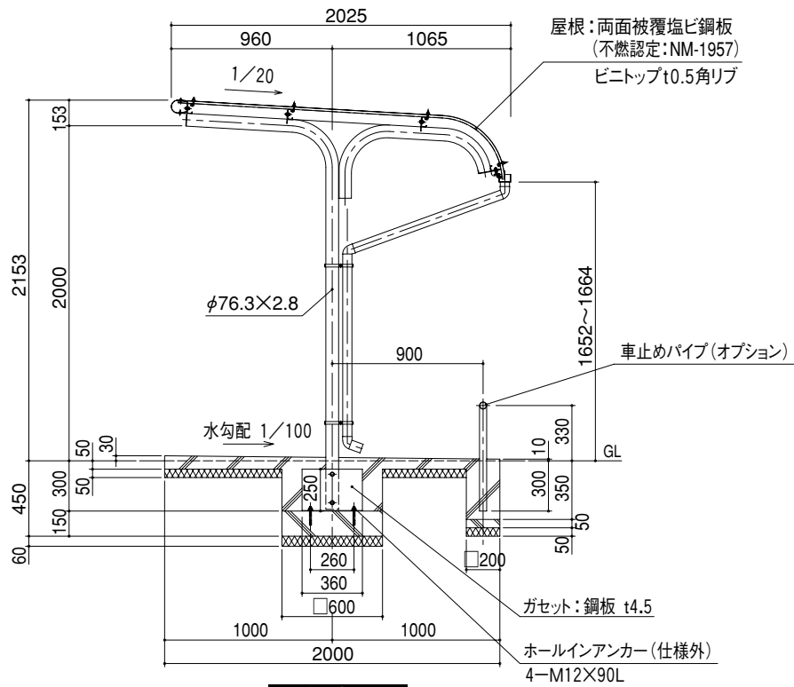
矩計図
