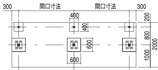
基礎伏せ図
