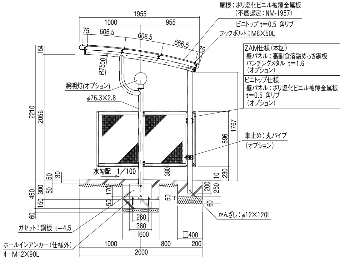
矩計図
